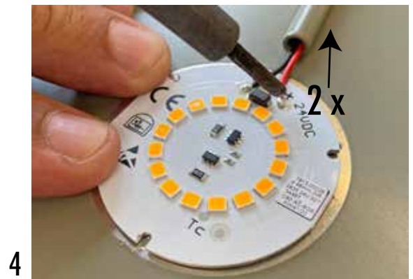
LötKolben - Soldering iron - Fer à souder - Saldatore - Soldador
